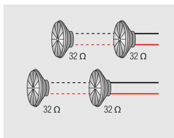
OPCIÓN PARA 4 ALTAVOCES OPTION FOR 4 LOUDSPEAKERS
